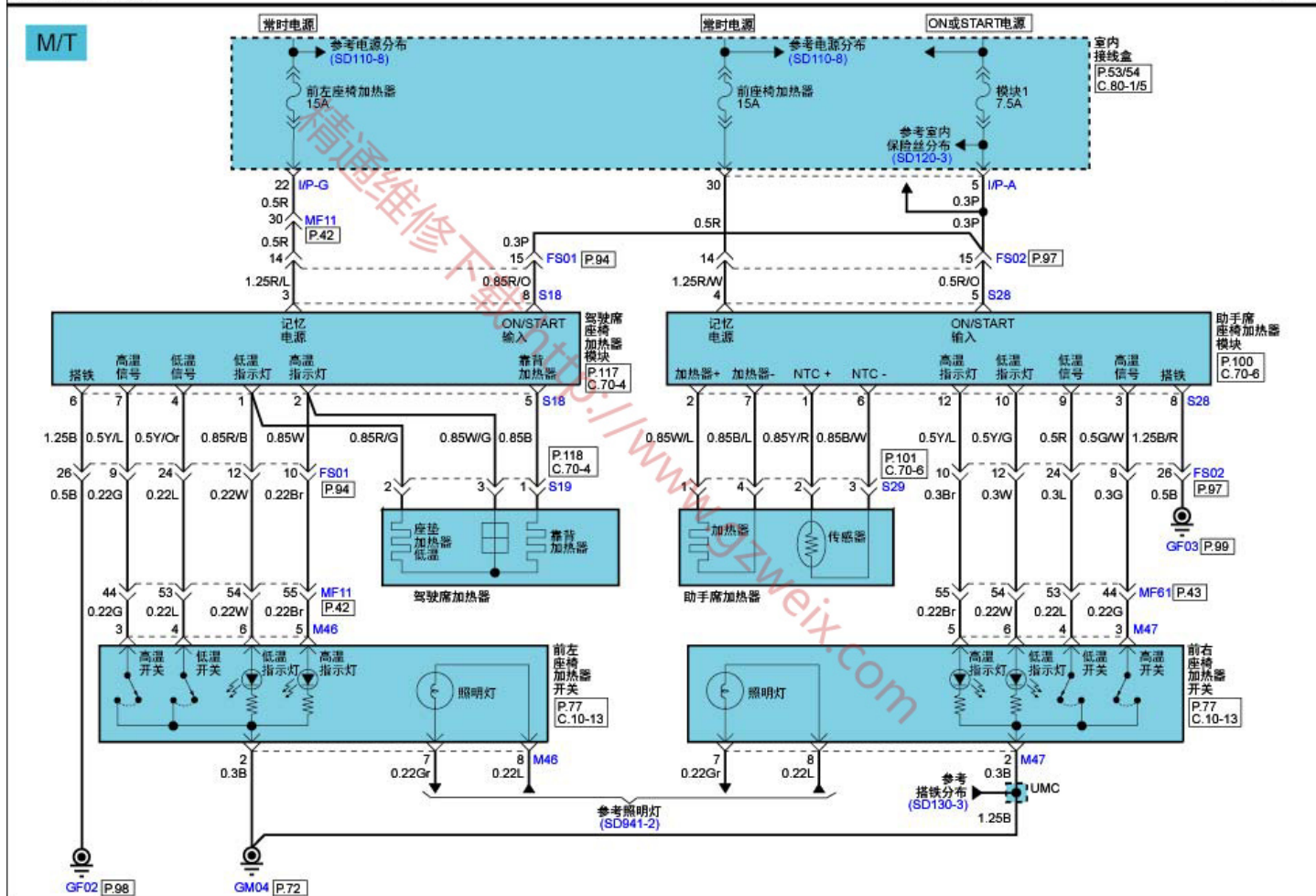
座椅加热器(1)
